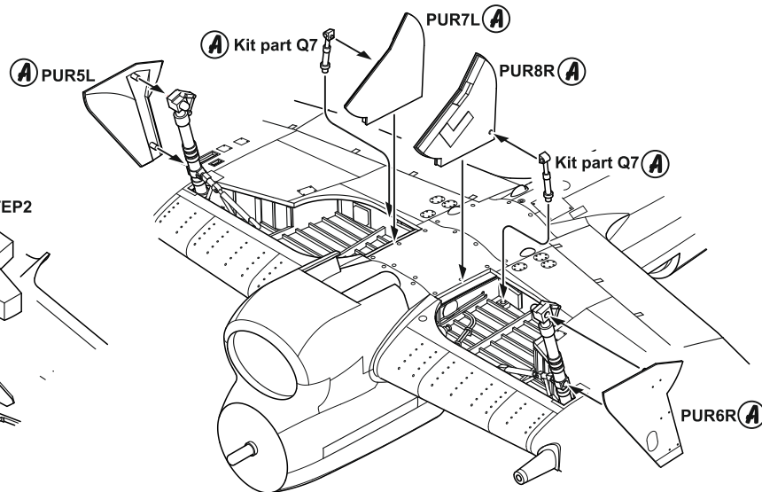
④ Montáž krytů podvozku / Mainwheel doors assembly
