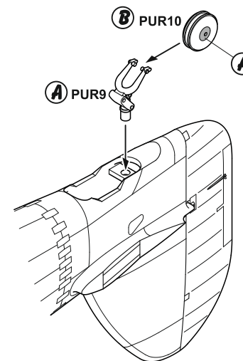
⑤ Sestavení ostruhy / Tailwheel assembly
